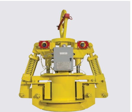
PINZA (VAAT)
